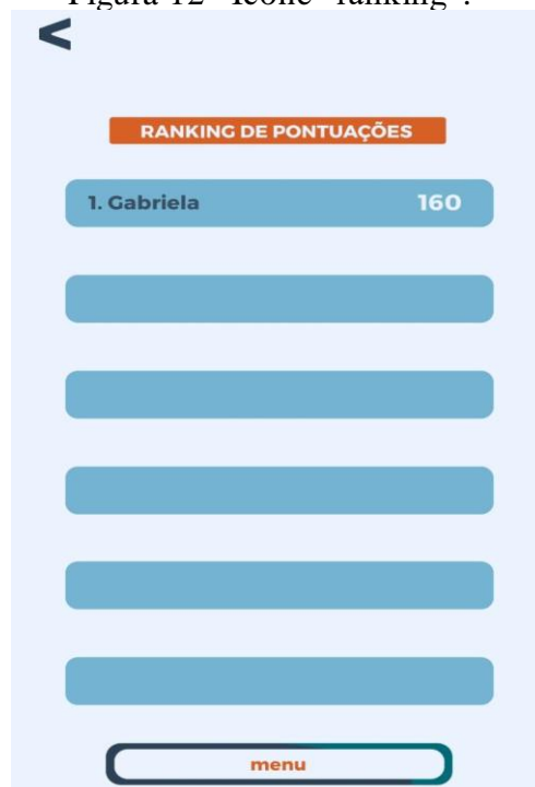
Figura 12 - Ícone “ranking”.
