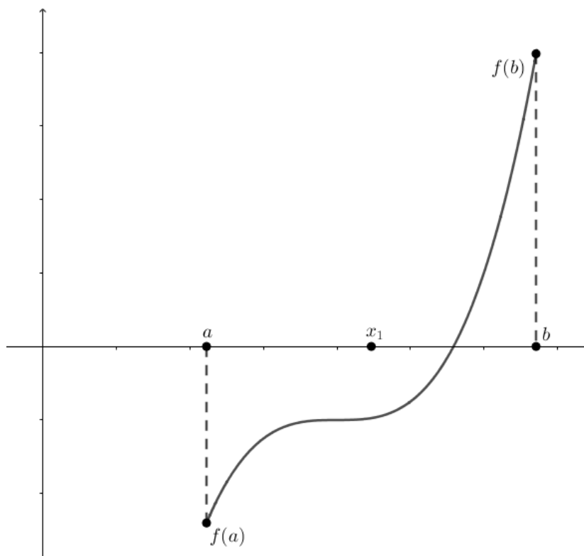
Figura 1 – Primeira iteração da bisseção
