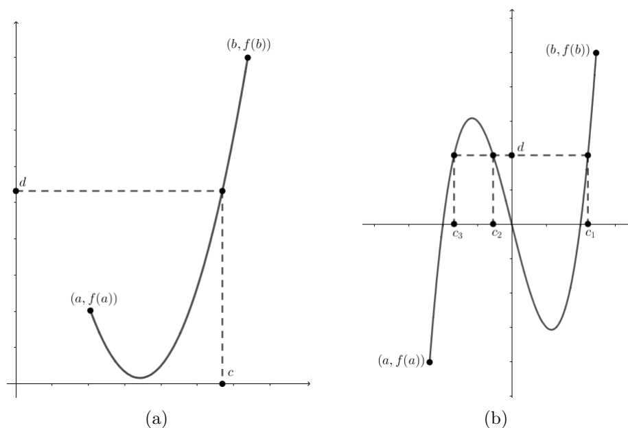
Figura 2 – Teorema do Valor Intermediário
