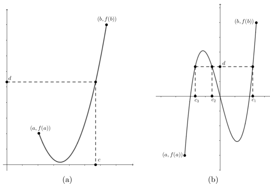
Figura 5 – Teorema do Valor Intermediário Caderno
