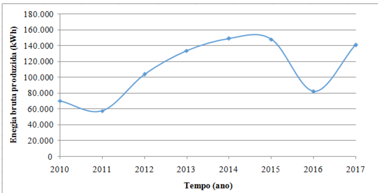
Figura 6 - Produção bruta de energia (kWh) ao longo do período de estudo.
