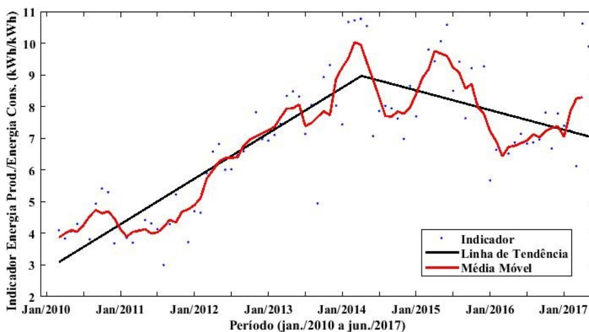
Figura 18 - Evolução do indicador de ecoeficiência “energia produzida/energia consumida (kWh/kWh)” no período 2010-2017.
